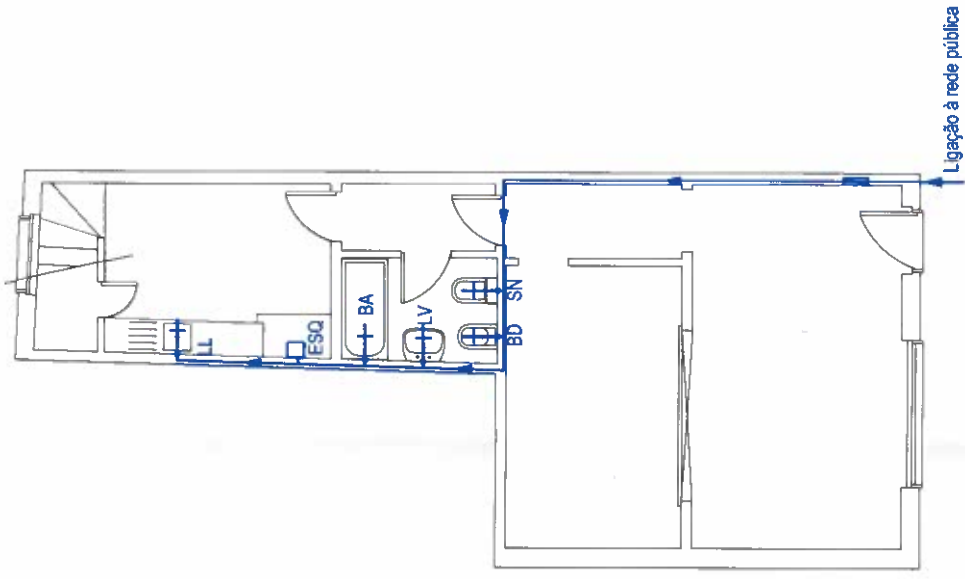
REDE DE ÁGUA FRIA
