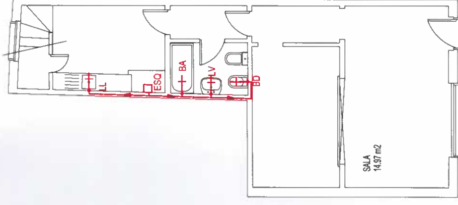
REDE DE ÁGUA QUENTE
