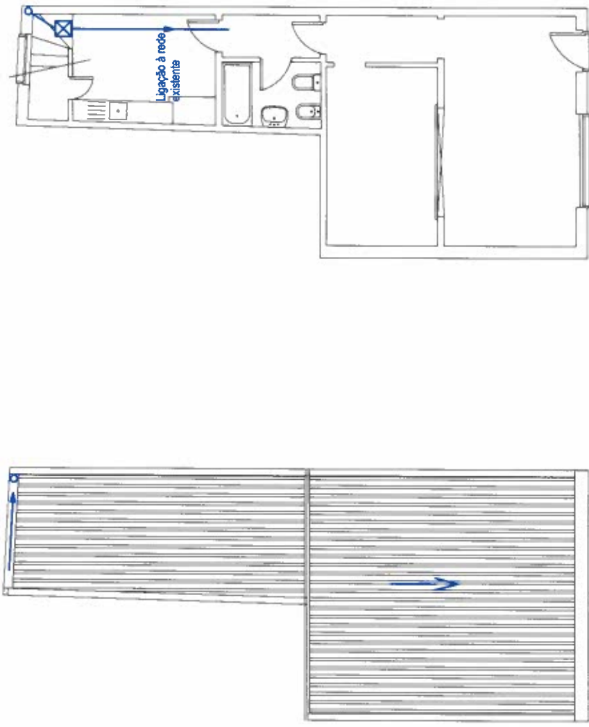
REDE DE DRENAGEM ÁGUAS PLUVIAIS
