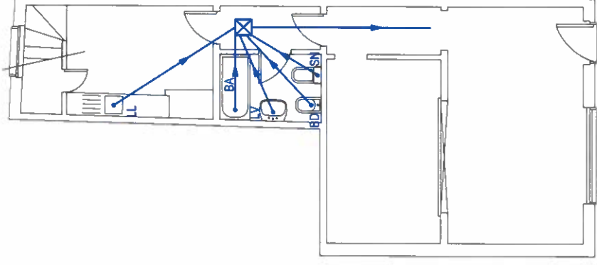
REDE DE DRENAGEM ÁGUAS RESIDUAIS DOMÉSTICAS
